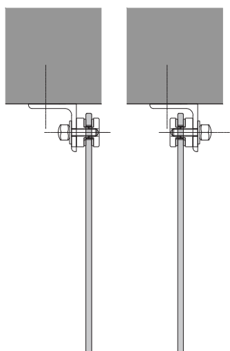
ŘEZ A
