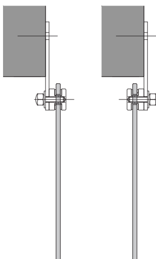
ŘEZ B
